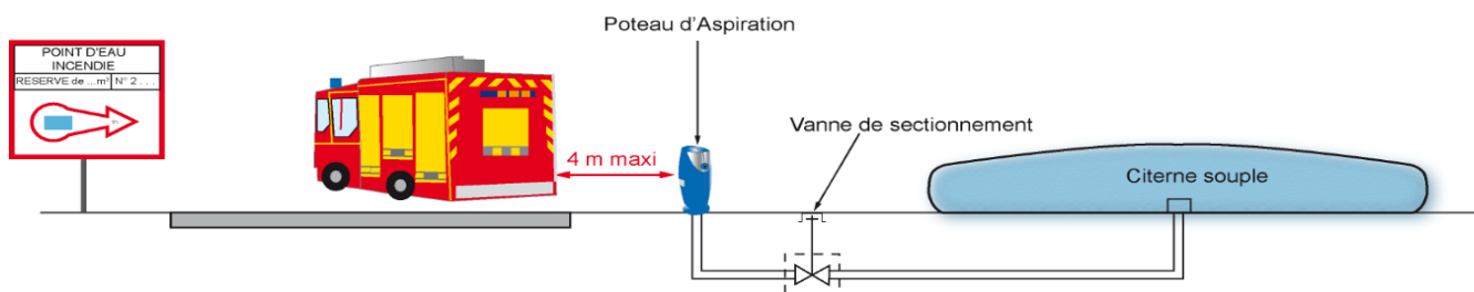
Citerne souple de 120 m³ équipée d'un Poteau d'Aspiration DN 100
